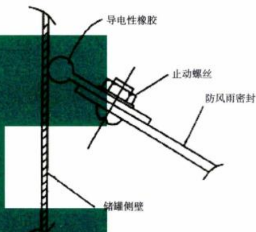
图8 防风雨密封与储罐侧壁的跨接
