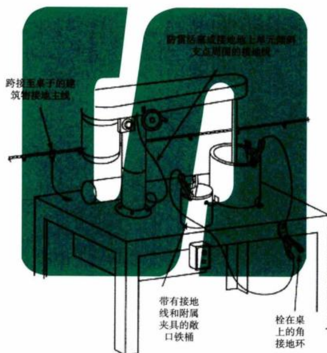
图C.6 小型设备的典型接地系统连接
