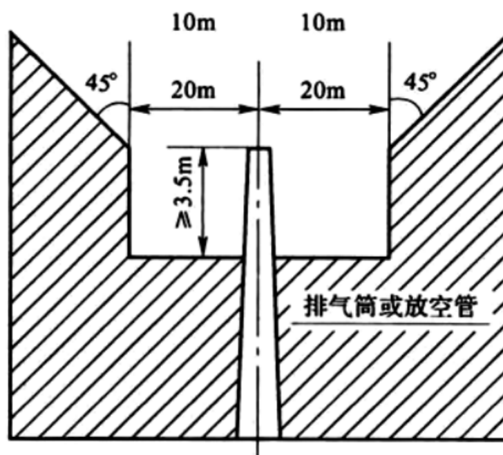
图 5.5.11 可燃气体排气筒、放空管高度示意图
