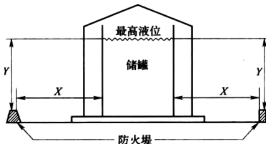
图 6.3.6 单储罐至防火堤内顶角线的距离
